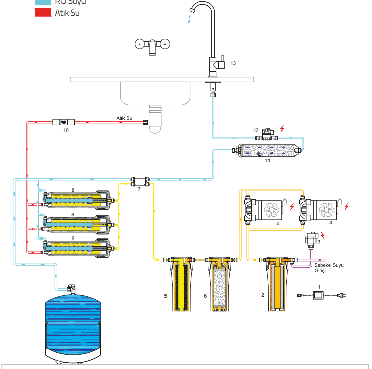
Şekil 2. RO Sistem Şeması
