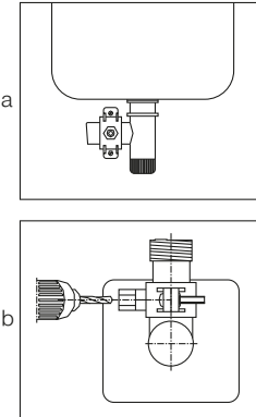
Şekil 7. Atık su bağlantısı
