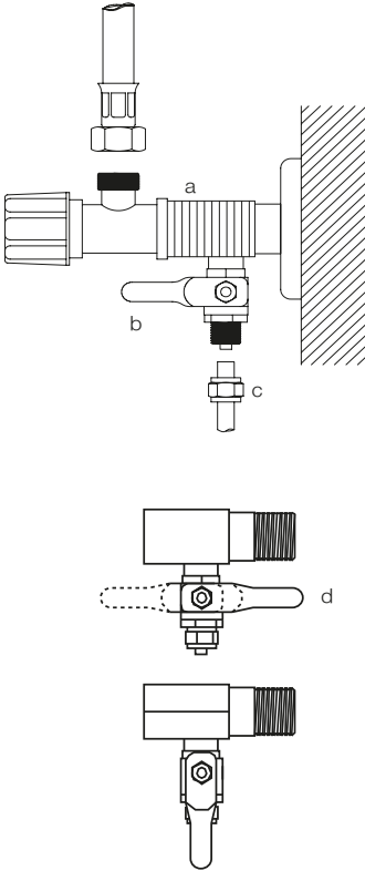
Şekil 5. Su bağlantı elemanları
